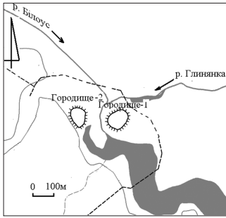
Рис. 1. Городища та річково-водна система в с. Малий Листвен.
